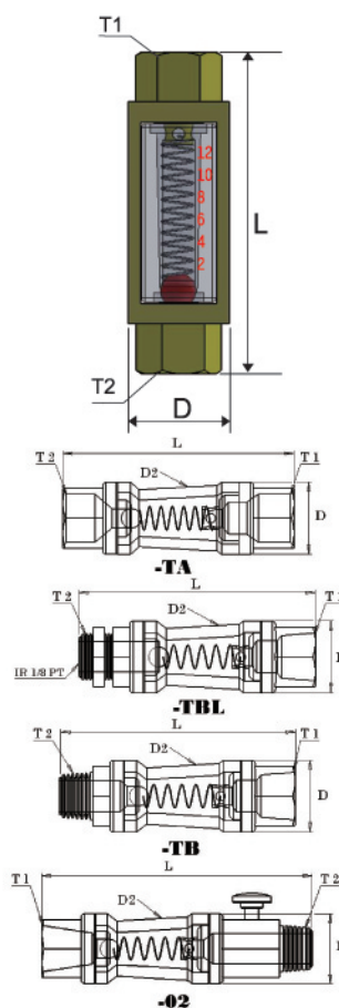
▲SK-01TBL 雙內牙(附螺母)
